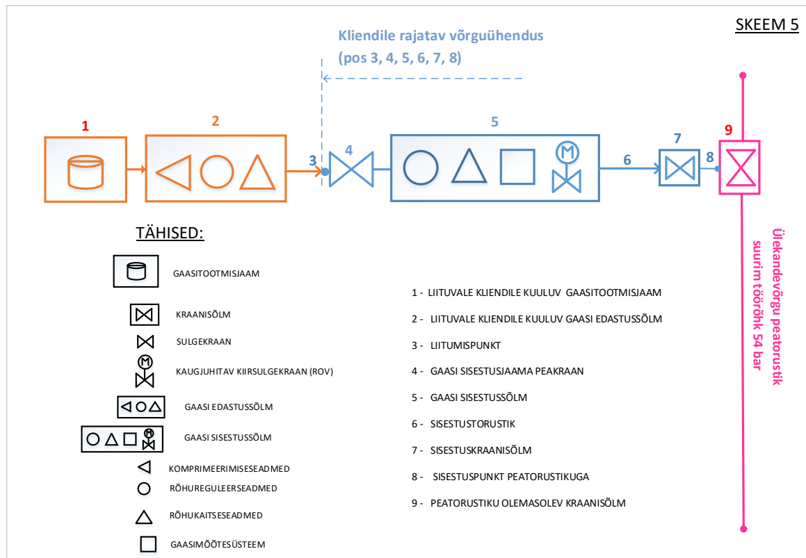
Joonis 5. Tootmissuunalise võrguühenduse näidisskeem
